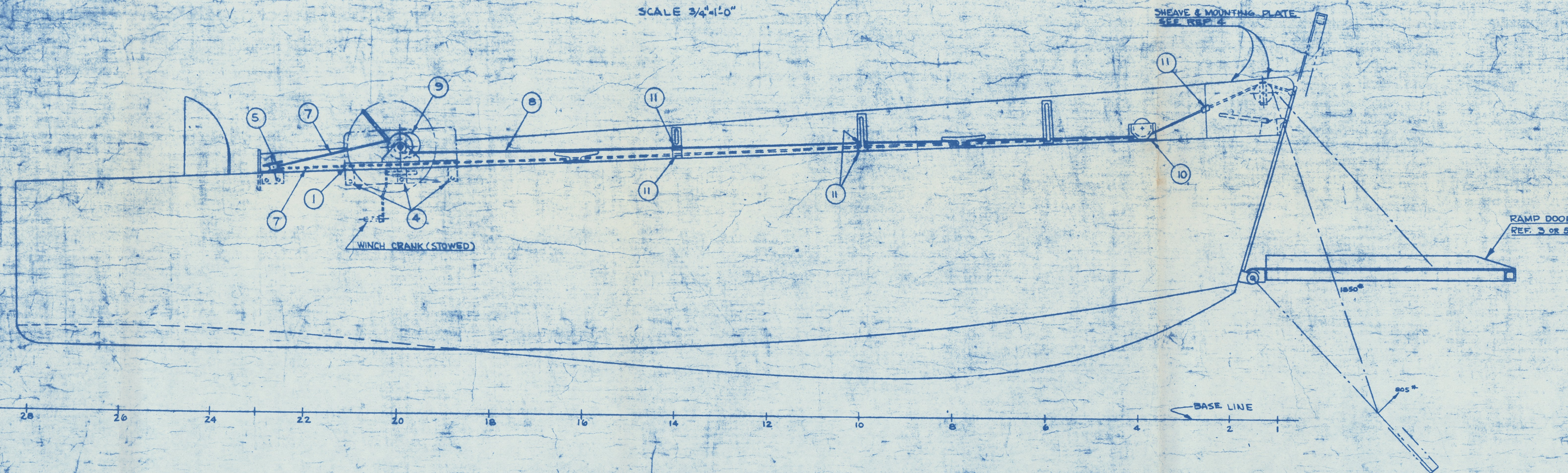
STARBOARD ELEVATION SCALE: 3/4" = 1'-0"
